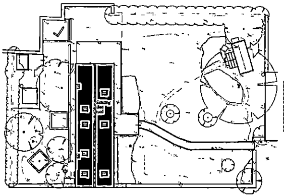
EXISTING SITE PLAN SCALE 1 : 200
